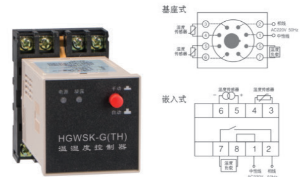
HGWSK-G(TH) 温湿度控制器
