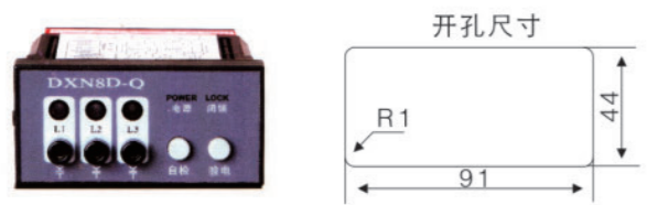
DXN8D-T(Q) 户内高压带电显示器(带自检、带验电)
