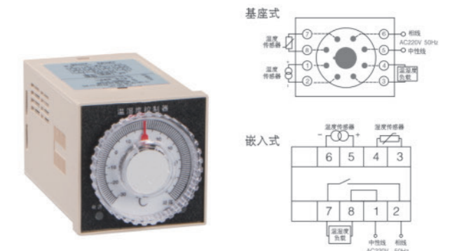
HGWSK-H(TH) 可调式温湿度控制器
