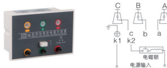
DXN-Q II型 高压带电显示器(验电型)
