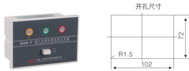
DXN-T(Q) I 高压带电显示器(提示型)
